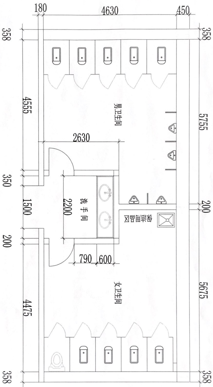
试制车间一层西侧公共卫生间平面布置图 (共2个)
