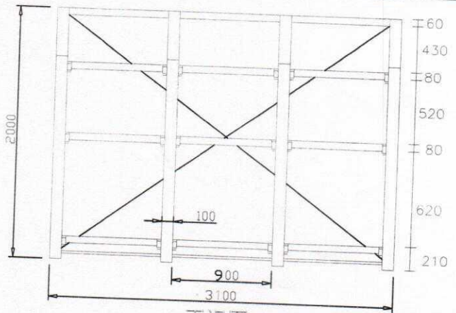
正视图
