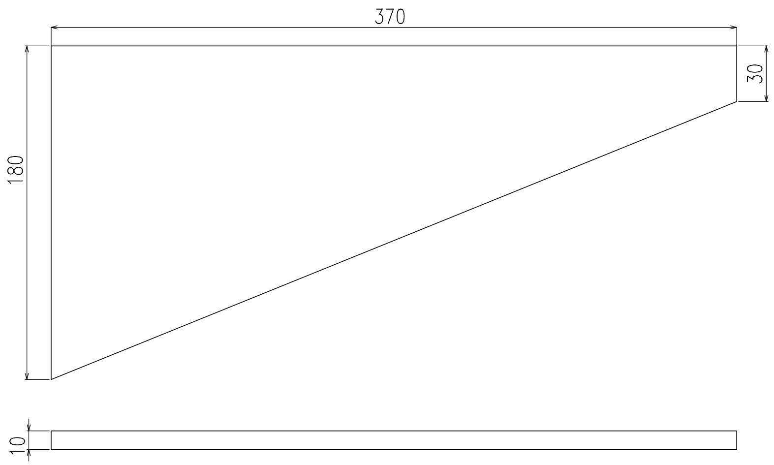
滚圆机设备延伸侧板，材质A3板，数量2个
