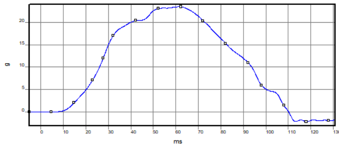
正面碰撞: 试验曲线
