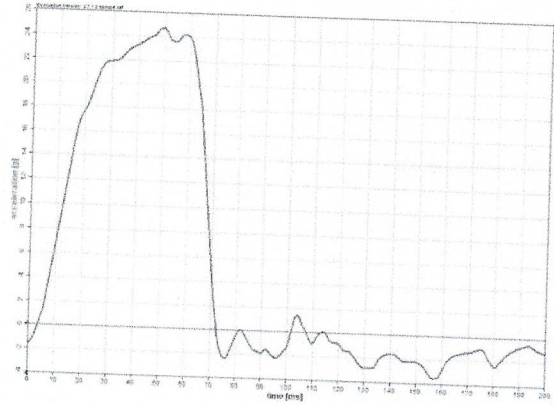
后面碰撞 b: 试验曲线
