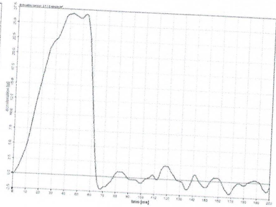
正面碰撞 b: 试验曲线
