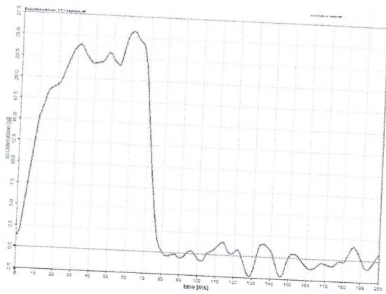
后面碰撞 a: 试验曲线
