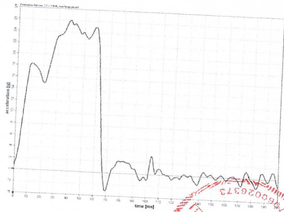
后面碰撞 b: 试验曲线
