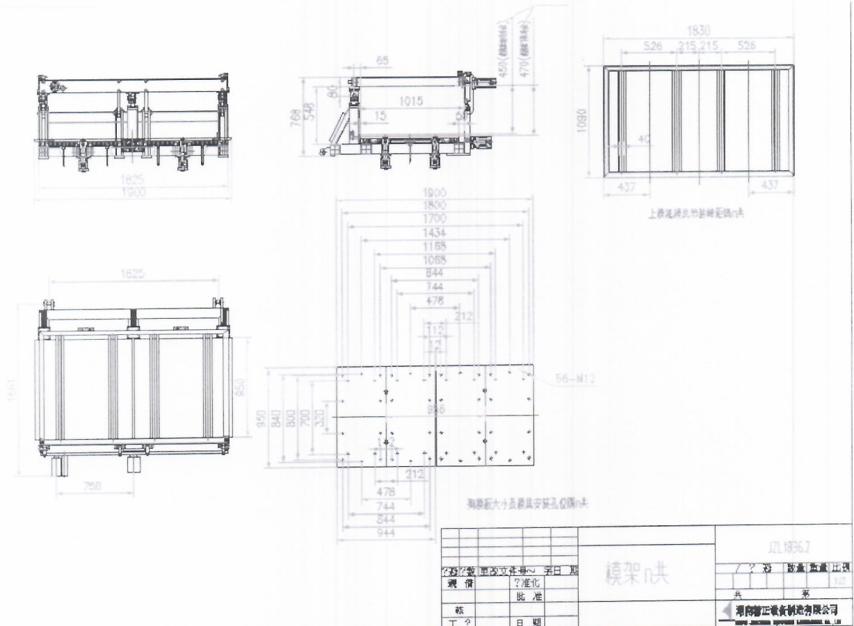
模架尺寸图
