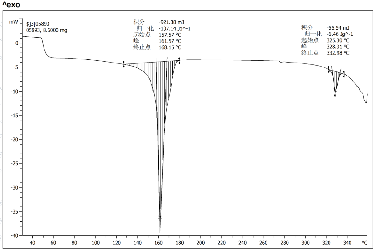
图 4 样品的 DSC 测试图
