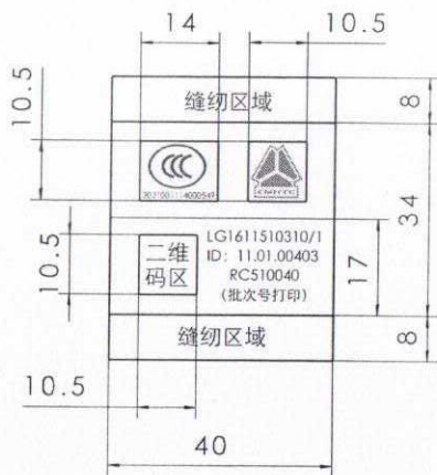
标识布局图
