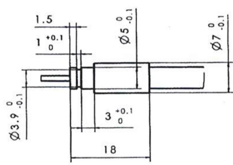
详图C
