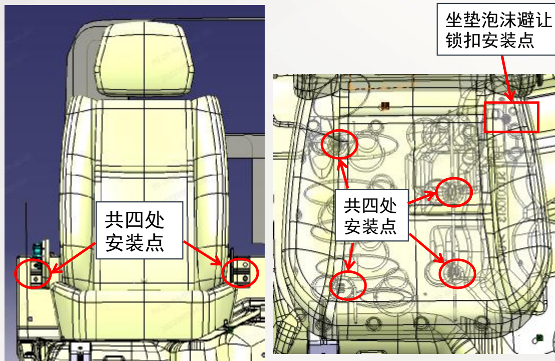
副驾座椅安装
