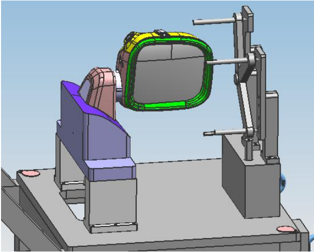
检具主体安装后视镜状态
