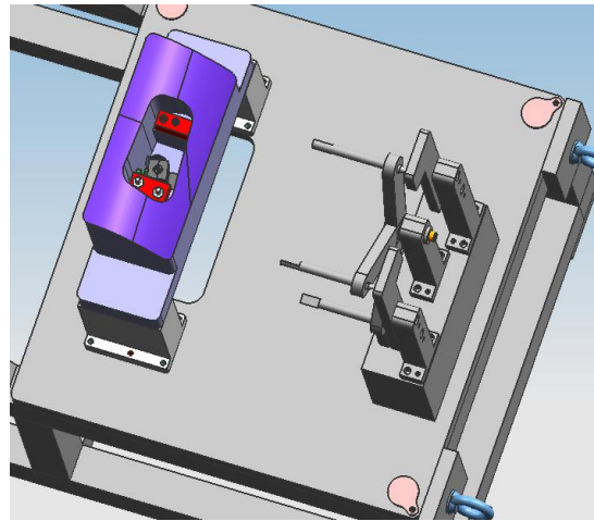
检具主体未安装后视镜状态
