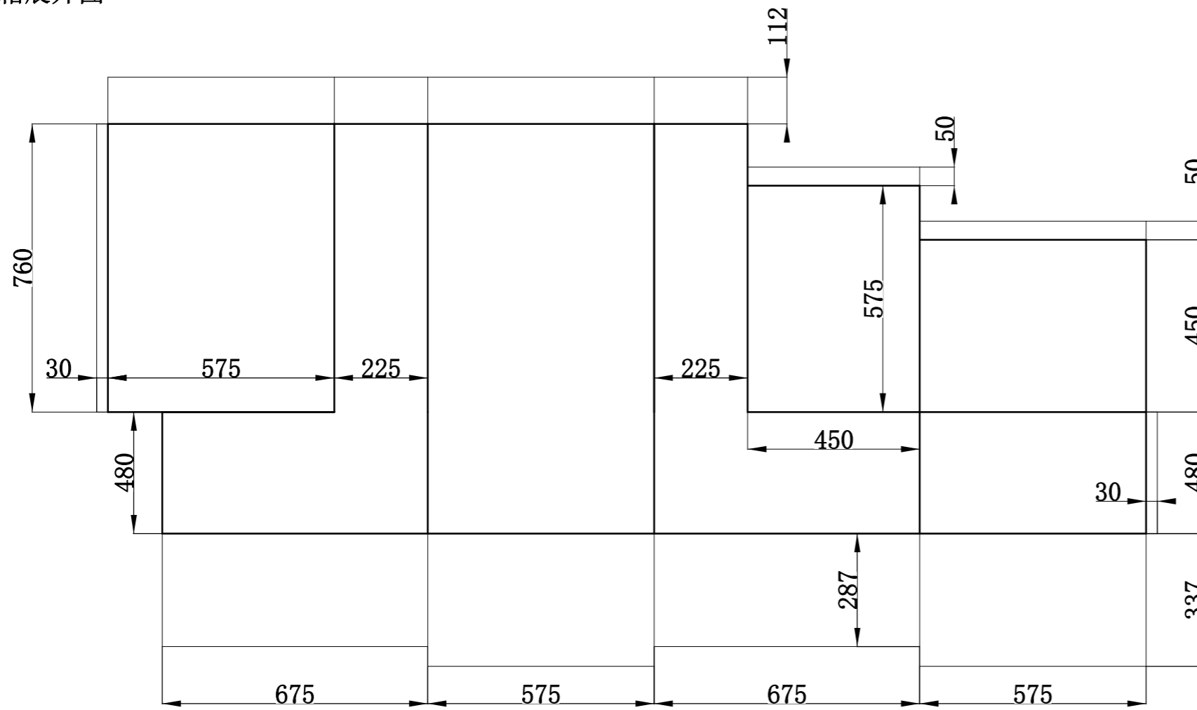
纸箱展开图
