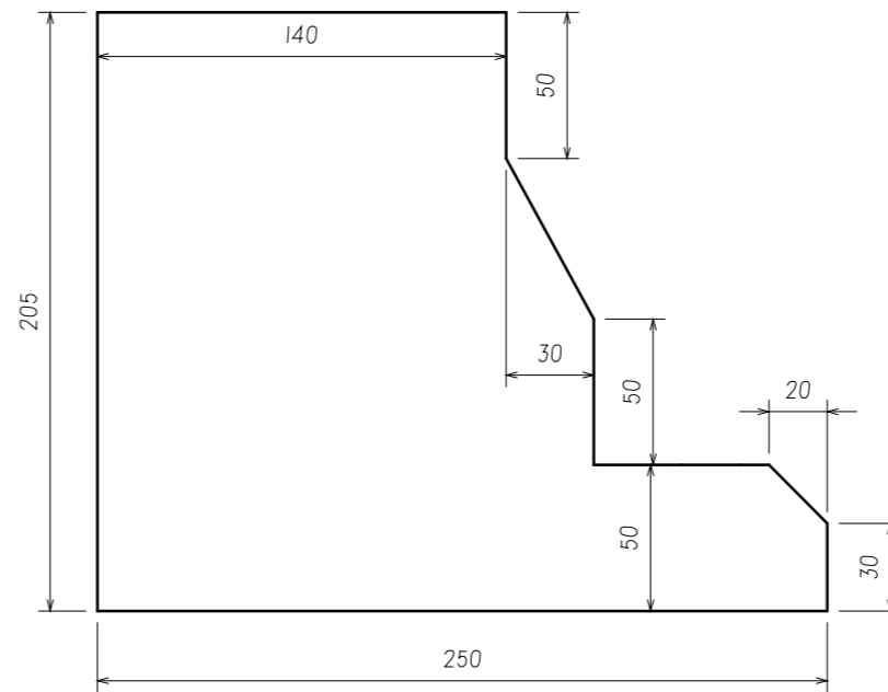
左视图 缩放: 1/2
