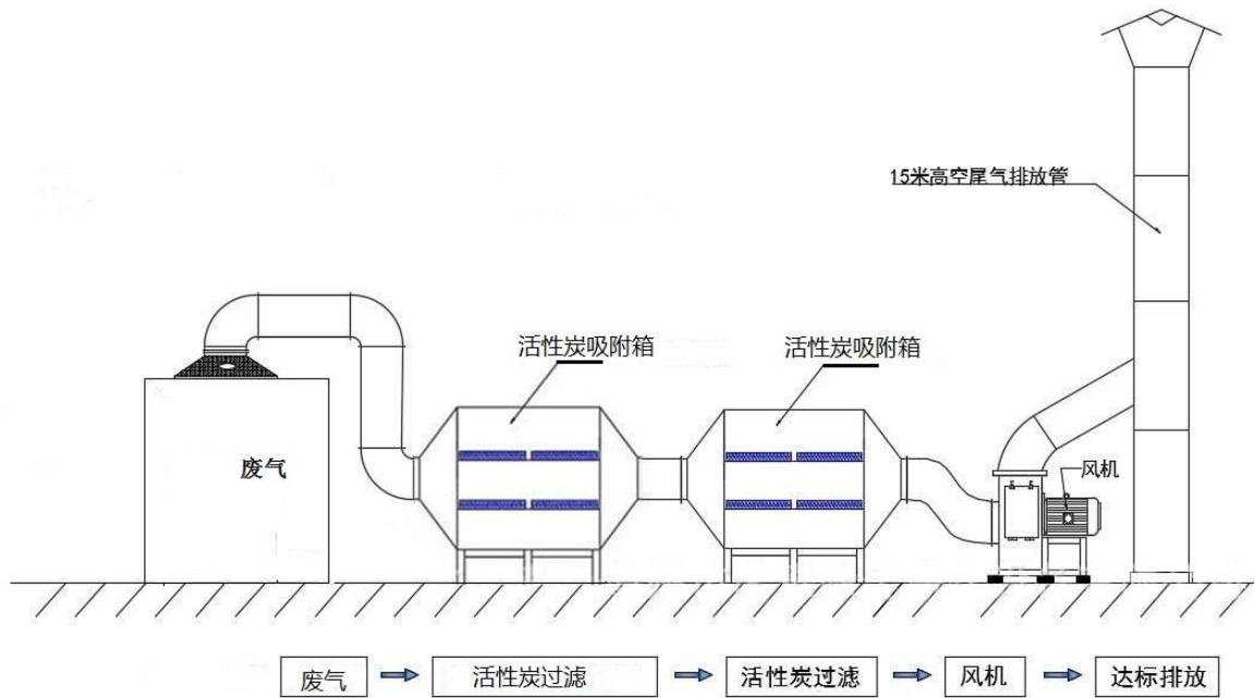
(废气处理工艺流程示图)
