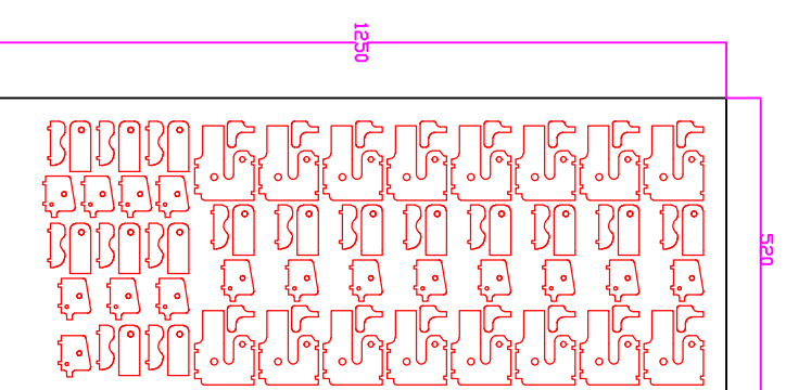
支架 材质: Q235/420/440/590 料厚: 5.0
