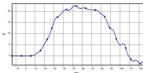
正面碰撞：试验曲线
