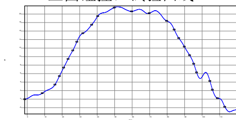
后面碰撞：试验曲线
