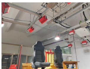
后面碰撞：试验照片
