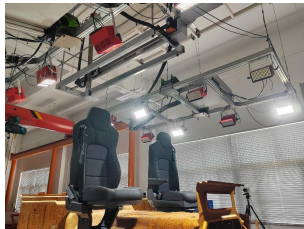
正面碰撞：试验照片
